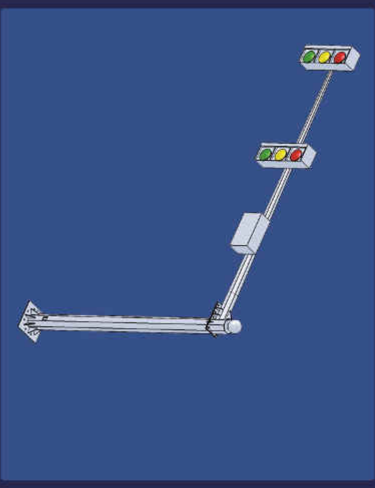
TRAFİK SİNYALİZASYON DİREĞİ / TRAFFIC SIGNALIZATION POLE
